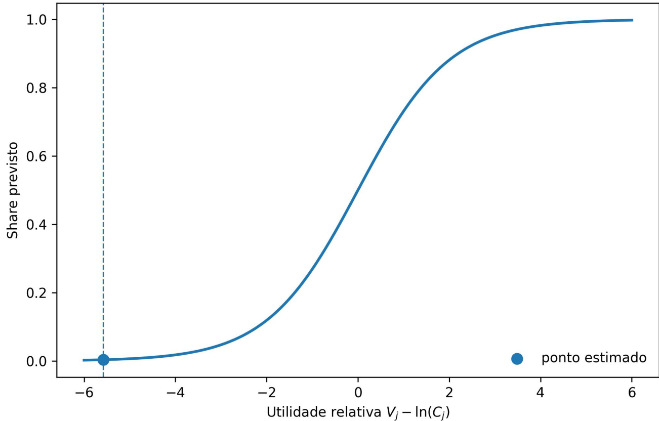
Curva clássica do logit - CornFlakes
